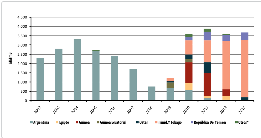
Gráfico N° 7. Origen de las importaciones de gas natural y gas natural licuado, año 2002 - 2013
