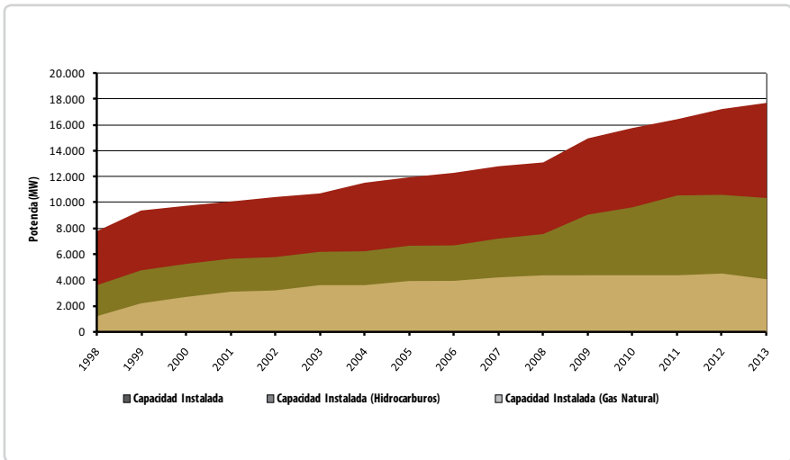
Gráfico N° 9. Evolución de la capacidad instalada de generación eléctrica, 1998 - 2013
