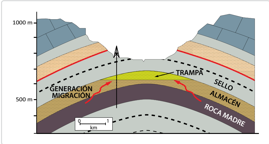
Figura N° 2. Estructura de un yacimiento convencional de hidrocarburo
