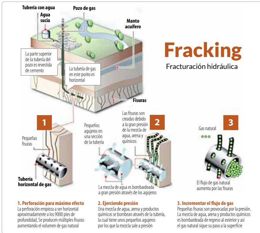
Figura N° 3. Proceso de fractura hidráulica
