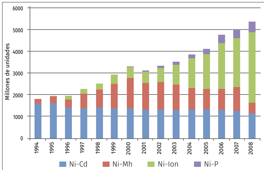
Gráfico N°2: Mercado mundial de baterías recargables
