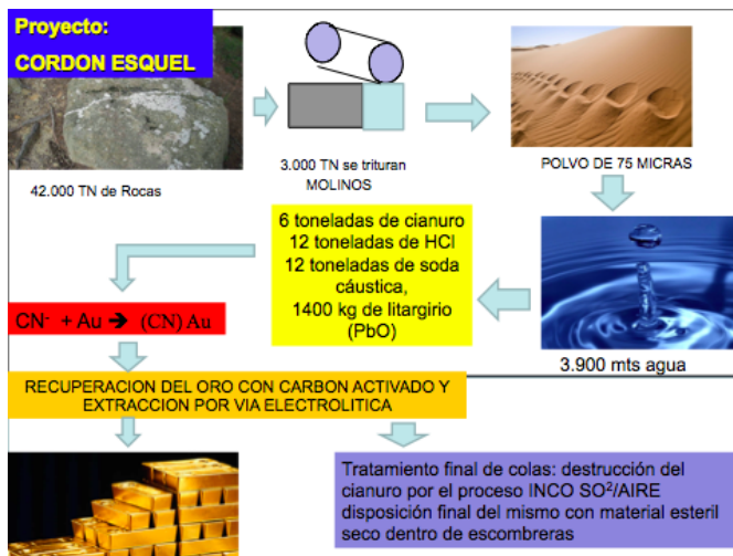
Figura 2: Modelo del proceso de explotación, a cielo abierto y con lixiviación con cianuro de sodio
